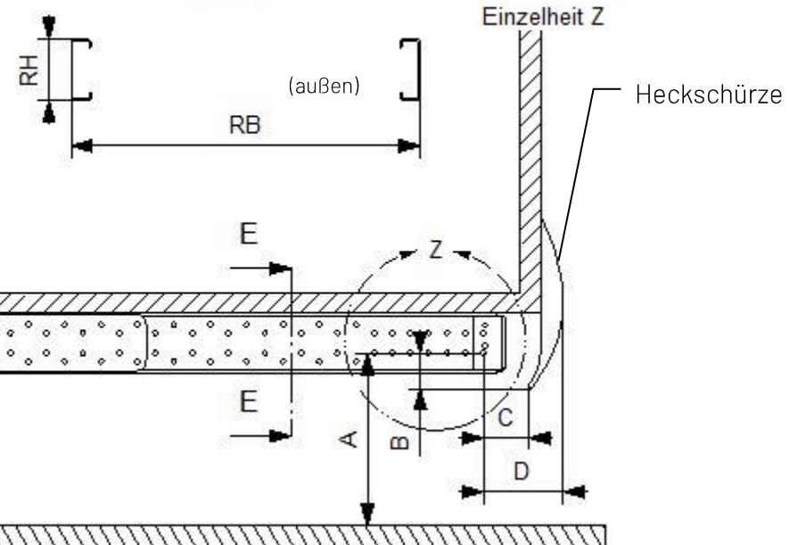
Schnitt E-E
